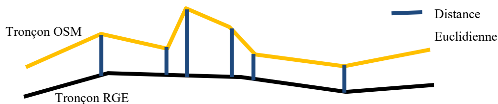
Schéma décrivant la méthode par distance euclidienne 32 (figure 8)
