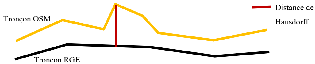
Schéma décrivant la méthode par distance de Hausdorff 32 (figure 7)
