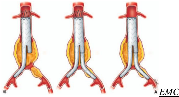
Figure 2 : Figure d'endoprothèse
