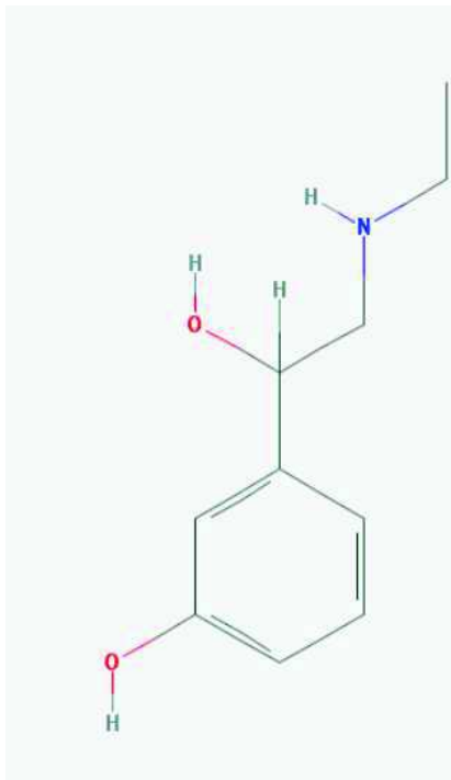
Figure 21 Etiléfrine (107)
