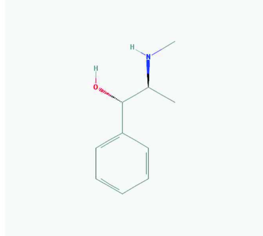
(1R, 2S)(+)-Pseudoéphédrine (85)
