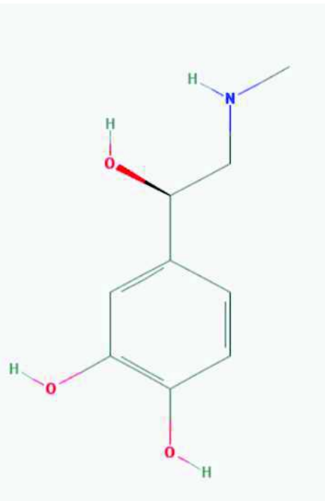
Figure 22 : Adrénaline (84)
