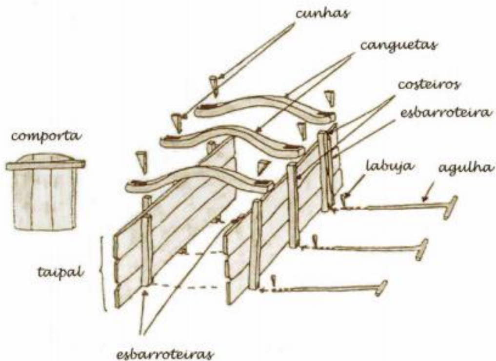
Parts of the rammed-earth frame-work. [Source: Parreira, Análise Sísmica de uma Construção em Taipas , p.7]
