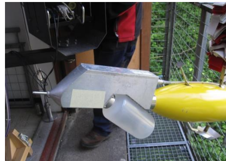
Figure 14 : Préleveur iso-cinétique de l'OFEV déployé lors des chasses du Rhône le 25 mai 2016 à la station hydrométrique de Chancy [HENRY E.]
