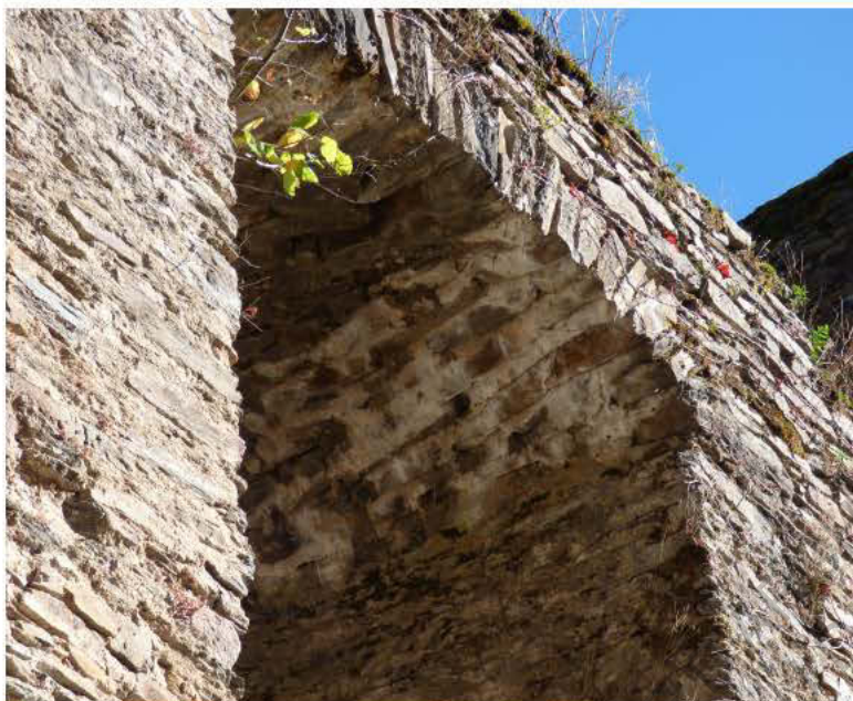
Bouchonnage d'une brèche (CdA)
