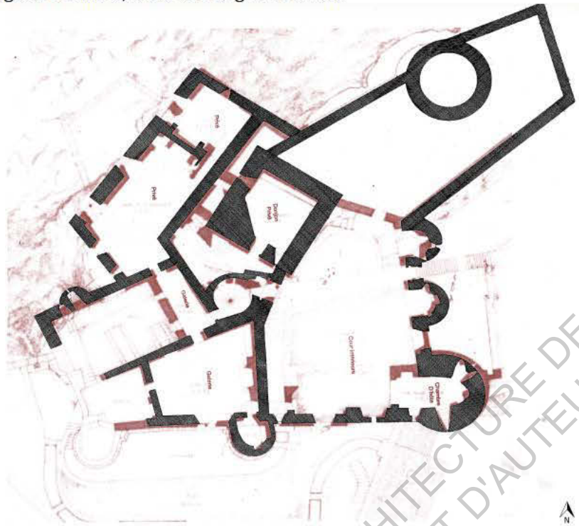
Plan du rez-de-chaussée mettant en valeur le projet de restauration (document retravaillé, sources château de Belcastel & STAP Aveyron)
