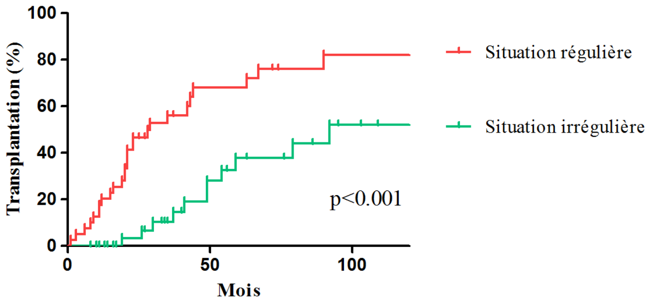
Figure 5 : Courbe d'incidence cumulée des patients transplantés par rapport à la mise en dialyse estimé par Kaplan Meier inversée ( p < 0.001 )
