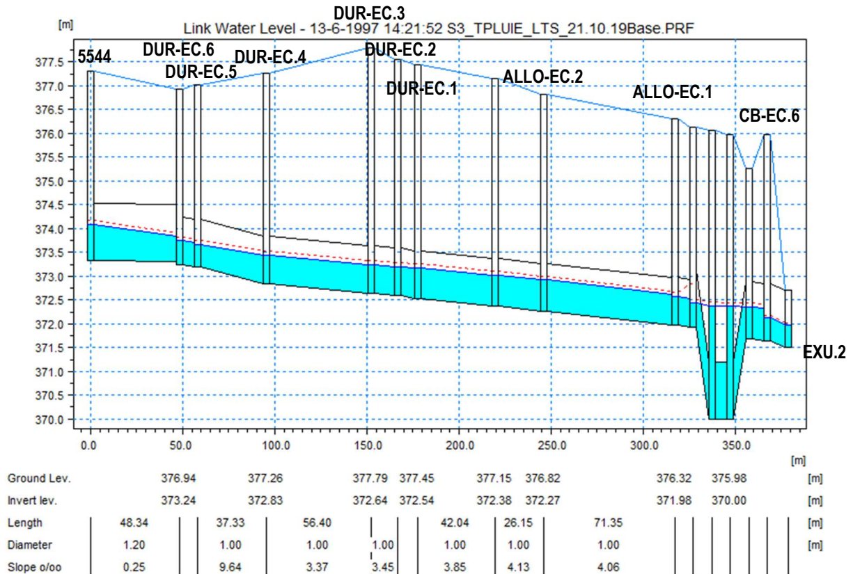
Figure 36 Hauteur d'eau dans les collecteurs de la rue Simon DURAND et Allobroges, solution VARIANTE, pluie du 13.06.1997
