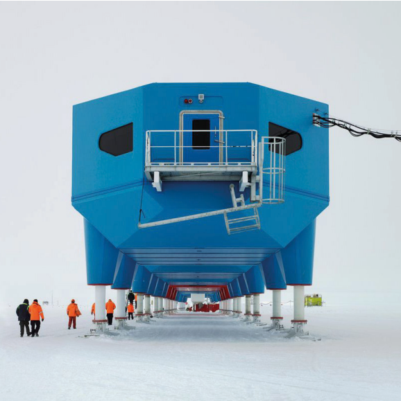
28. La base anglaise est surélevée pour faire face à l'accumulation de la neige
