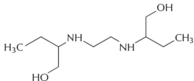
Figure 21 : structure chimique de l'éthambutol 27 .
