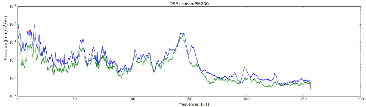
FIGURE 4.9 – Densité spectrale de puissance de la poutre du point métrique 200 de la campagne 2017
