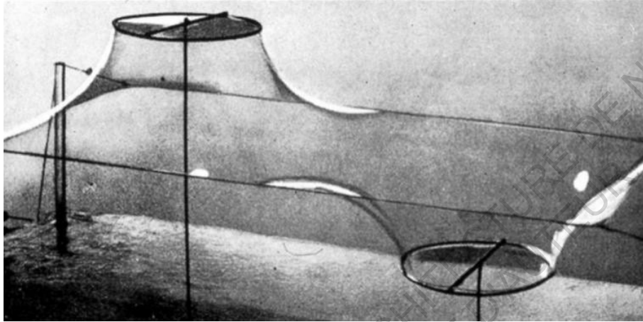
Maquette en bulles de savon Source : parcolympique.qc.ca
