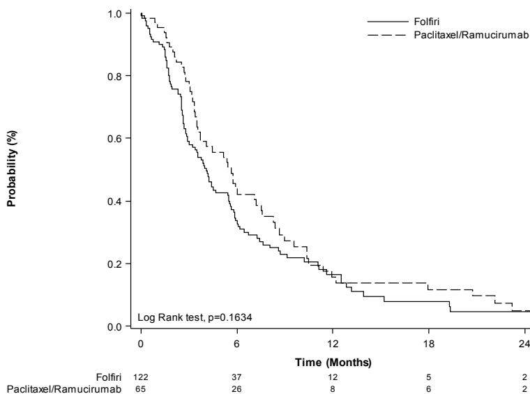
Figure 2 : Survie sans progression L2 par traitement (bras PR et FIRI)
