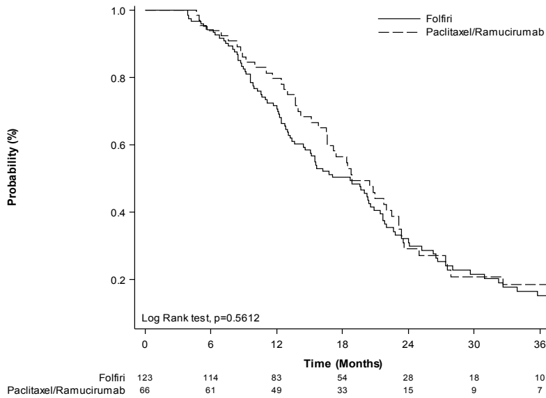
Figure 1 : Survie globale L2 par traitement (bras PR et FIRI)
