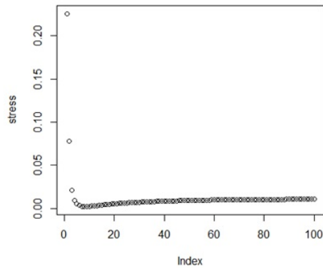
FIGURE 3.7 – Stress de la reconstruction des pseudo-comptes de E. coli
