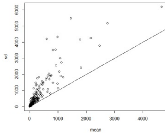
FIGURE 3.4 – Dispersion des comptes de l'analyse 16S en fonction de la moyenne observée ( n = 842 ). La droite représente la relation attendue sous l'hypothèse que les comptes suivent une loi de Poisson
