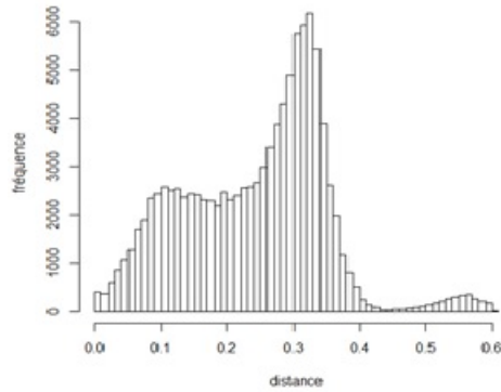
FIGURE 3.5 – Histogramme des distances Unifrac pondérées entre échantillons de E. coli
