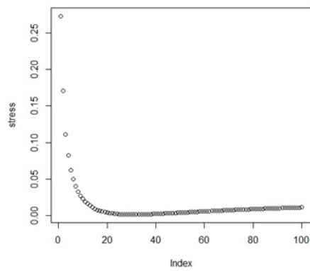
FIGURE 3.8 – Stress de la reconstruction des pseudo-comptes de 16S
