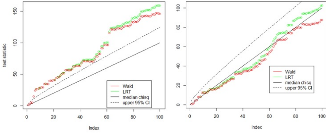
FIGURE 3.10 – Statistique de test en fonction de la dimensionnalité pour l’association entre microbiote intestinal et BMI (gauche : 16S, droite : E. coli)
