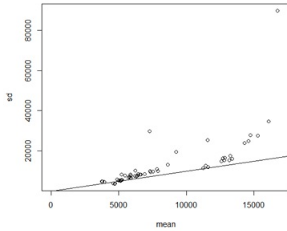
FIGURE 3.3 – Dispersion des comptes de E. coli en fonction de la moyenne observée ( n = 56 ). La droite représente la relation attendue sous l'hypothèse que les comptes suivent une loi de Poisson
