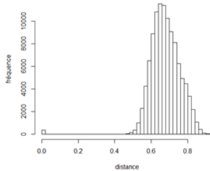
FIGURE 3.6 – Histogramme des distances Unifrac pondérées entre échantillons de l'analyse 16S
