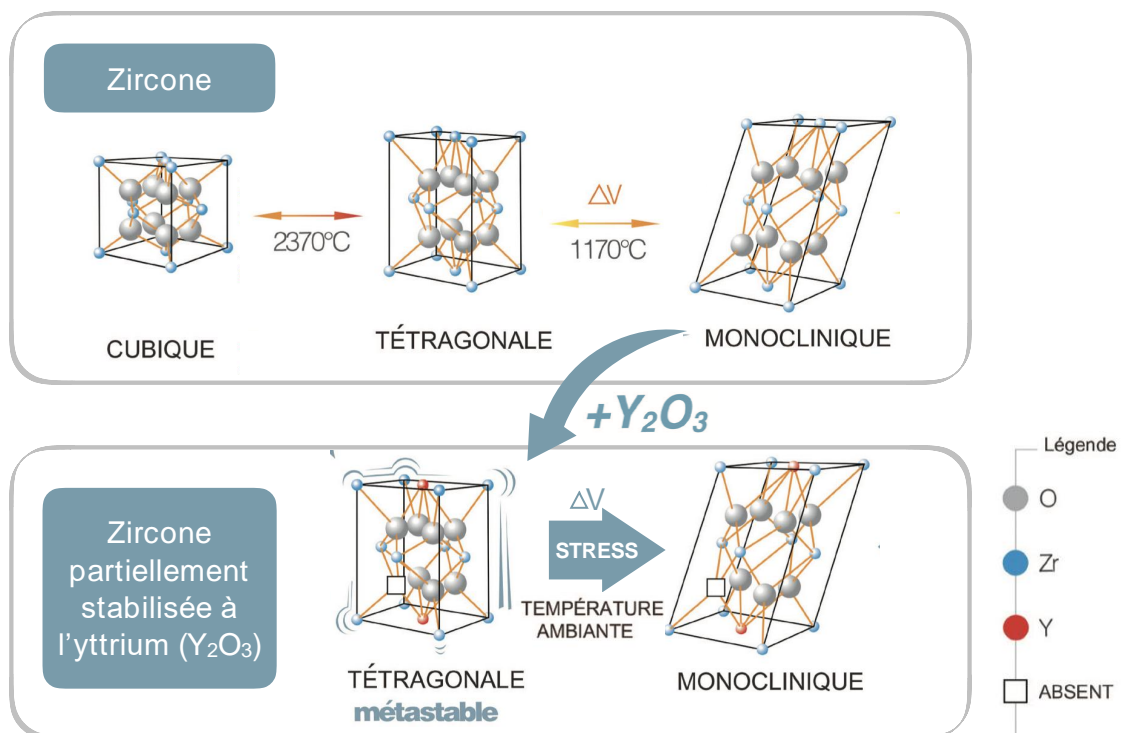
Figure 7 : Figure des trois formes cristallines de la zircone selon l'apport thermique (en haut) et du passage, à température ambiante, de la forme tétragonale métastable à monoclinique de la zircone partiellement stabilisée à l'yttrium après un stress mécanique notamment (en bas)
