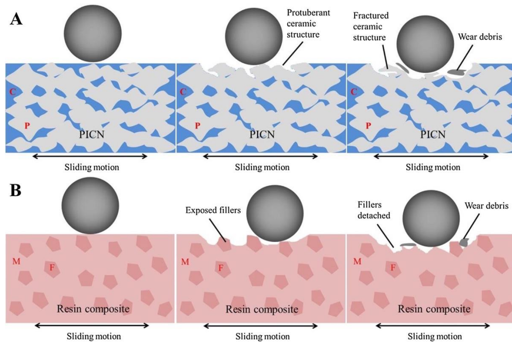
Figure 20 : Représentation schématique de l'usure et du procédé et dégradation de VitaEnamic (en A) et de résine composite à charges dispersées (en B). En A : le C désigne la portion résineuse et le P désigne la portion inorganique. En B : M désigne la matrice organique et F désigne les charges dispersées.
