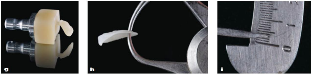
Figure 18 : Photographies d'une table tops en PICN (VitaEnamic) usinée en faible épaisseur (0,2 mm)
