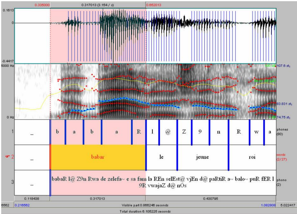
Figure 1 : exemple d'une représentation acoustique de la parole analysée sous PRAAT (de haut en bas : l'oscillogramme, le spectrogramme, et les trois « tires d'intervalle » pour annoter phonétiquement) – Goldman 2006
