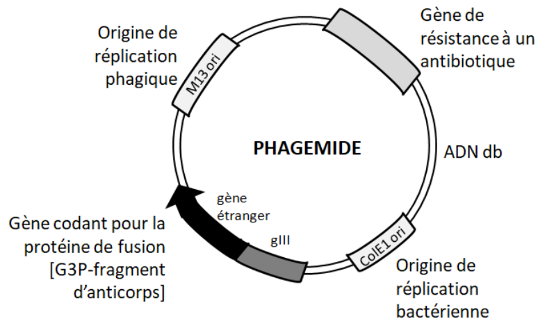
Figure 29 : Vecteur phagemide
