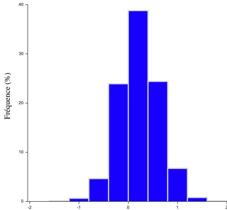
Figure 3. Simulation de données selon une loi normale. Moyenne = 0.2 ; Ecart-type = 0.4
