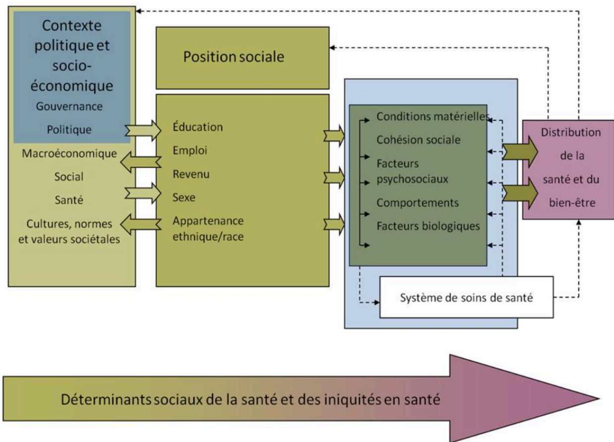
Figure 2 : modèle CDSS
