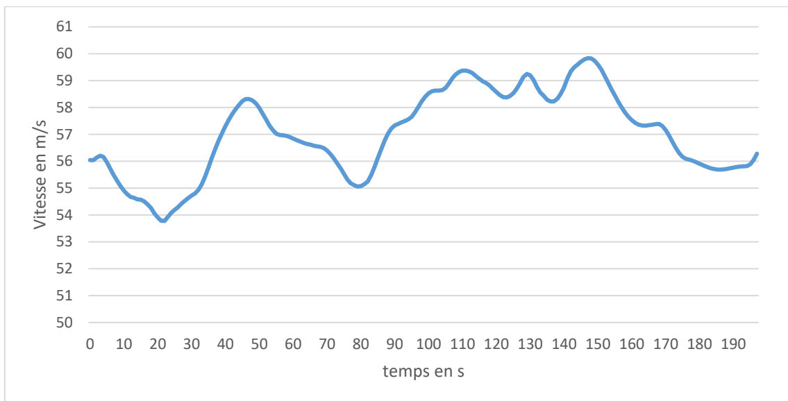
Figure 22 : Evolution de la vitesse de l'avion lors d'un vol LiDAR
