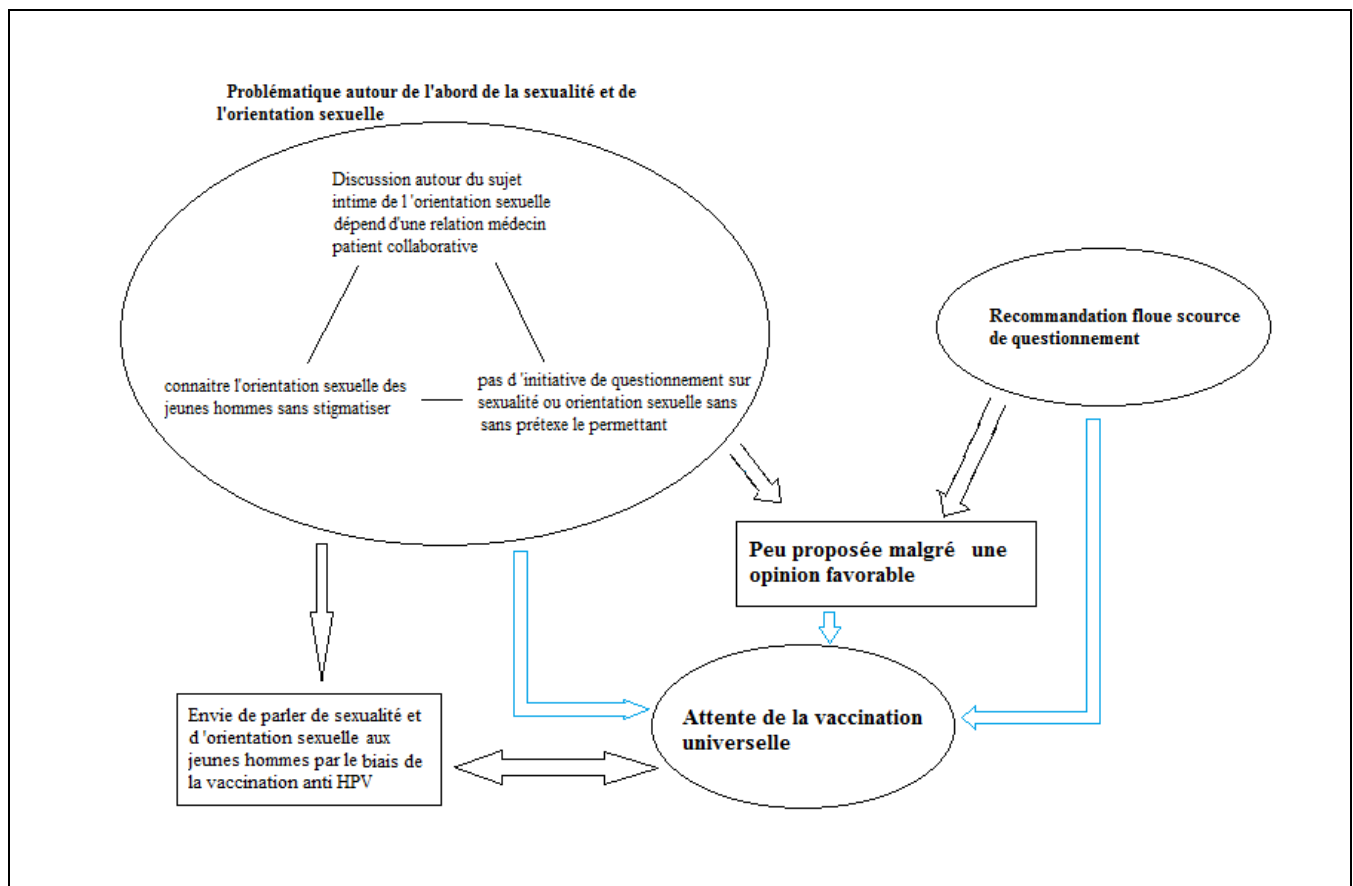
Figure 4 : Modélisation
