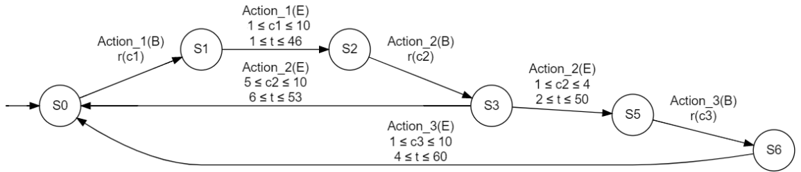
FIGURE 2 – Un AT avec la syntaxe de Timed k-Tail. Les transitions correspondant au début d'un événement ont leur symbole accolé d'un « (B) » et une horloge est réinitialisée ( r(c_1), r(c_2), \dots ). Les transitions correspondant à la fin d'un événement ont leur symbole accolé d'un « (E) », une vérification de la valeur de l'horloge de l'événement et une vérification de l'horloge globale t .
