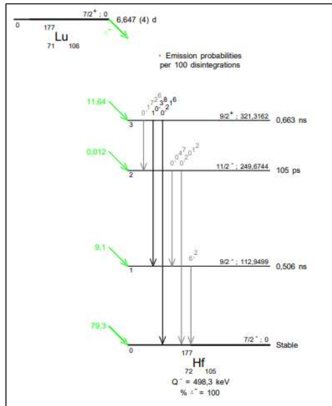
[Figure 12] - Schéma de désintégration du 177 Lu, d'après LNHB, CEA. (52)
