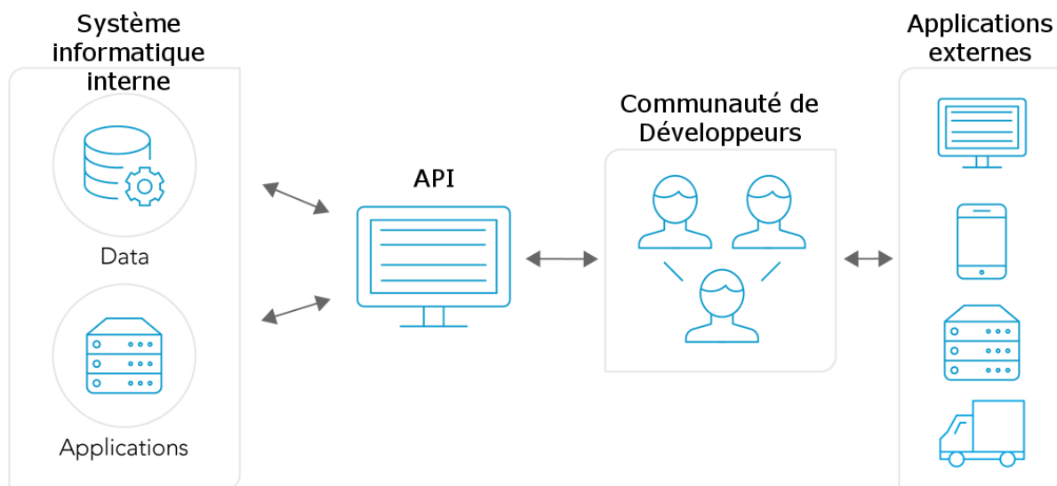
Figure 23 : Fonctionnement d'une API (d'après API Management Developer Portal from Software AG)
