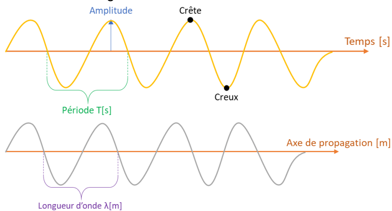
Figure 2: Les grandeurs caractéristiques d'une onde.
