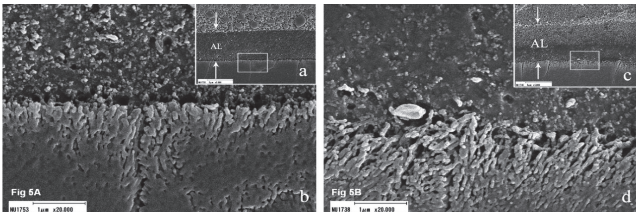
Figure 10 : Images représentatives au microscope électronique à balayage de l'interface adhésif-émail. AL: Couche adhésive Grossissement * 20,000 ; Figure (a): Scotchbond Universal appliqué en MR. (b): Scotchbond Universal appliqué en SAM(20).
