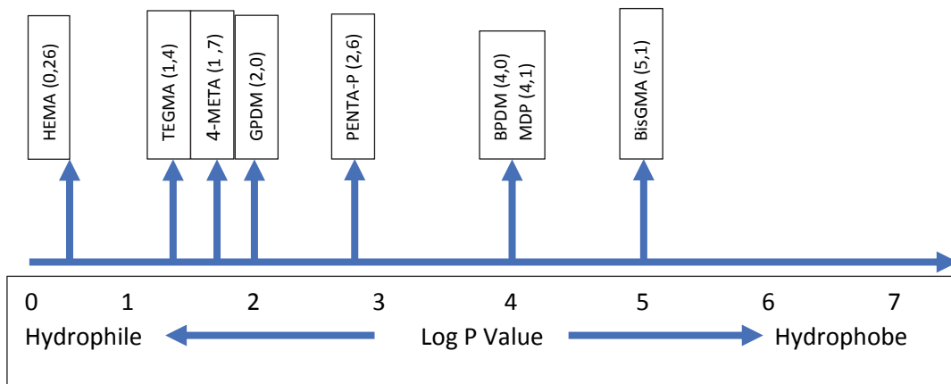
Figure 6 : Classement relatif des monomères en fonction de leur propriétés hydrophile / hydrophobe (13)
