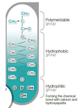
Figure 8 : schéma moléculaire de 10-MDP
