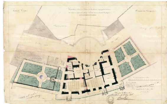
Figure 33 - Réparations à faire au château de Montferrier acquis par la commune et destiné à renfermer la mairie, les écoles communales et le presbytère : [plan d'ensemble du rez-de-chaussée] / dressé par l'architecte soussigné [Corvetto]. Montpellier, 5 mai 1845.
