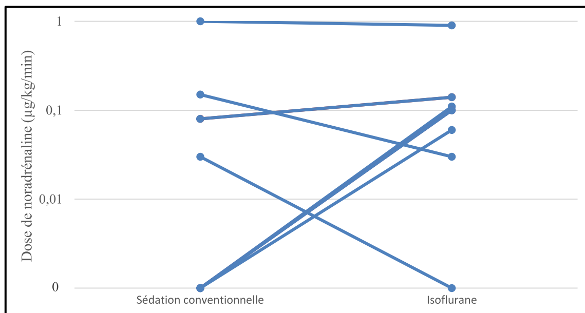
Figure 4 : Variation des doses de noradrénaline pour chaque patient
