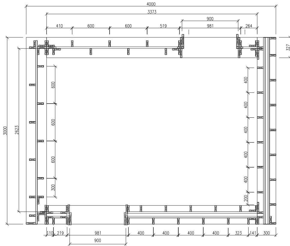
◀ 59 - Plan du prototype d'ossature bois à trame dédoublée - Ech. 1/50° - ▶ 60 - Coupe et élévation de l'ossature à entraxe 40 cm - Ech. 1/50° -
