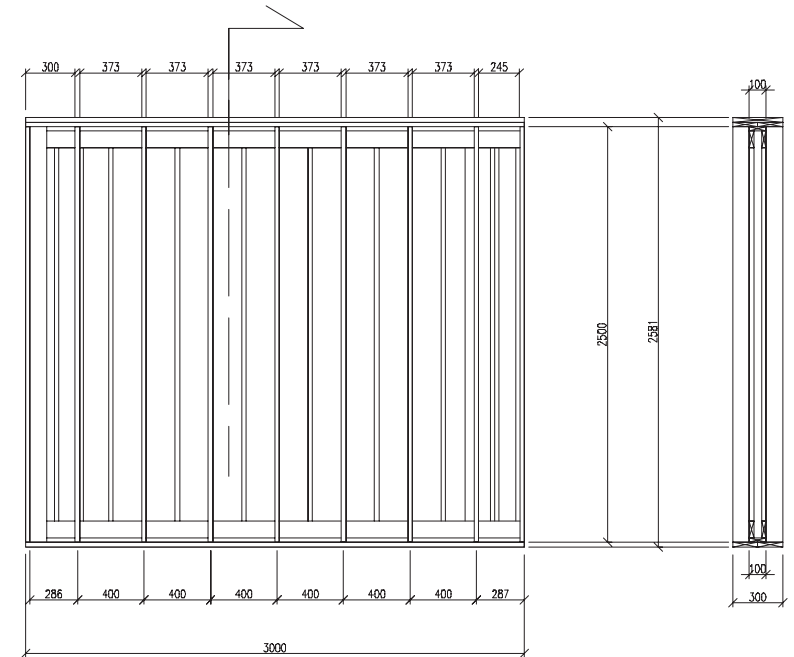
◀ 59 - Plan du prototype d'ossature bois à trame dédoublée - Ech. 1/50° - ▶ 60 - Coupe et élévation de l'ossature à entraxe 40 cm - Ech. 1/50° -
