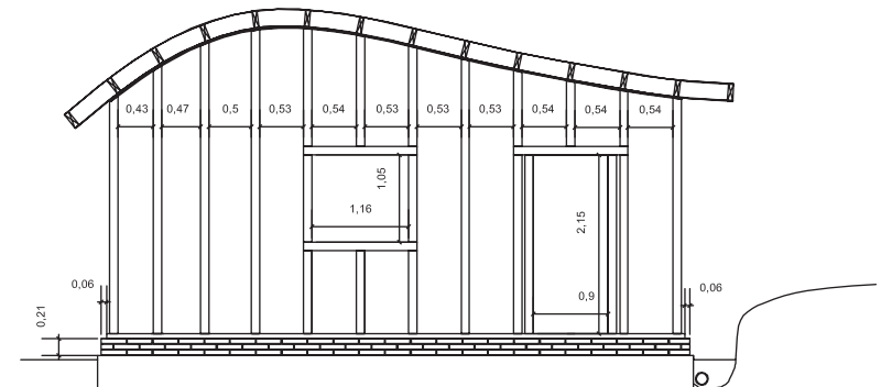
► 31 - Elévation Est de l'ossature principale. - Ech. 1/100° -
