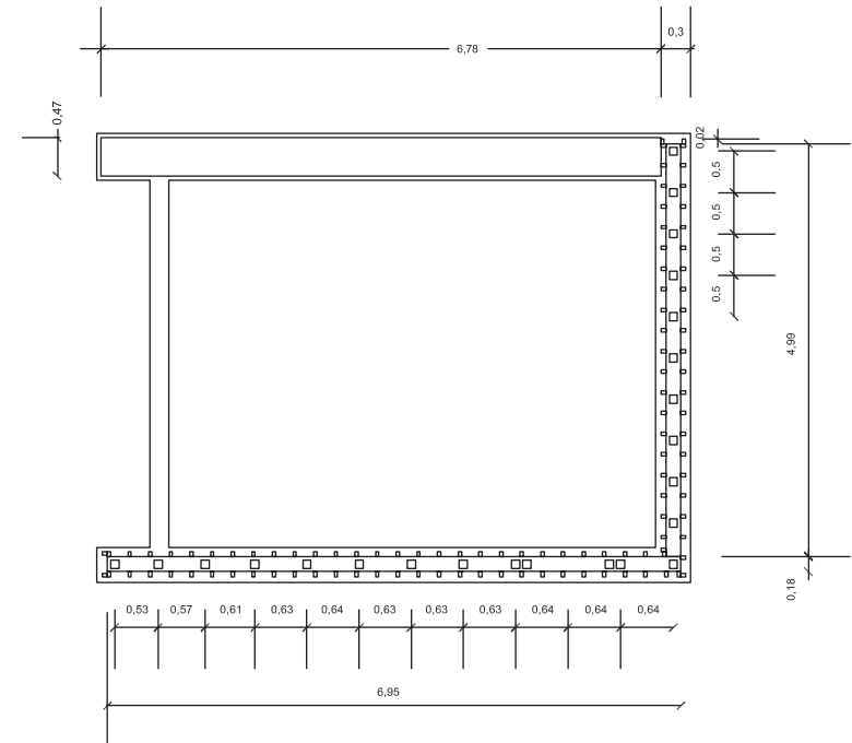
► 30 - Plan de l'ossature principale - Ech. 1/100° -
