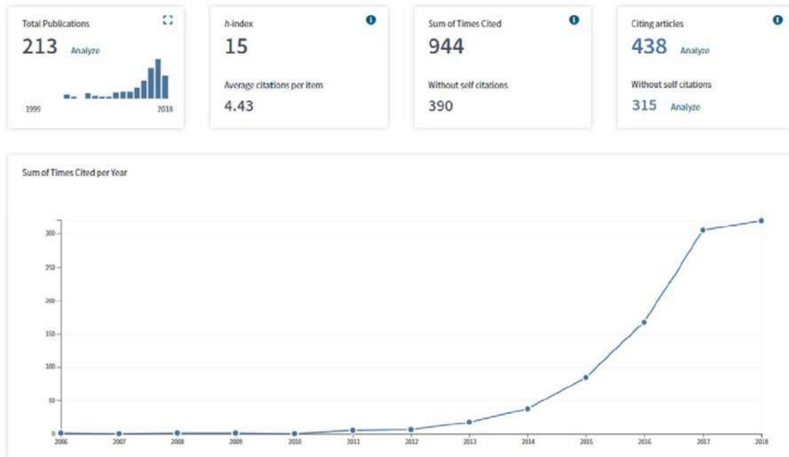
Figure 4 : résultat de la recherche du terme « aquaponics » dans la base de données Web Of Science ressortant le nombre de publications contenant ce mot clé (tiré de Yep and Zheng, 2019)
