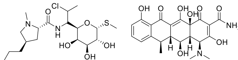
Figure 16 : Structures chimique de la clindamycine (à gauche) et de la doxycycline (à droite).
