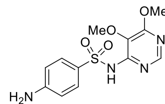
Figure 14 : Structure chimique de la sulfadoxine.
