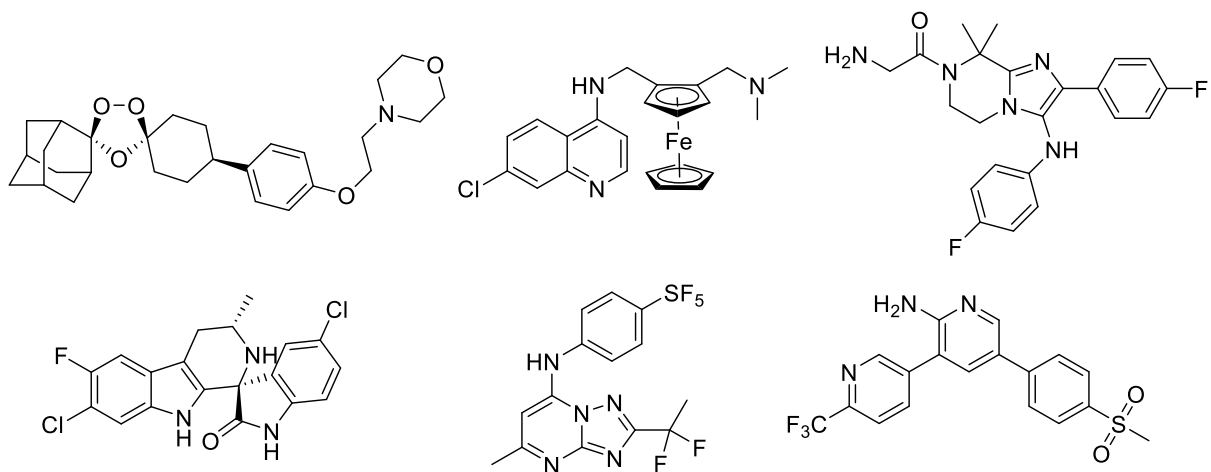
Figure 20 : Structures chimiques, de la gauche vers la droite, de l'artéfénoméle, de la ferroquine et du ganaplacide (en haut) et de la cipargamine, du composé DSM265 et du composé MMV048 (en bas).
