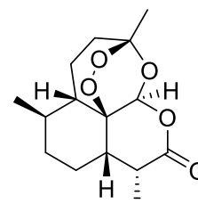
Figure 18 : Structure chimique de l'artémisinine.
