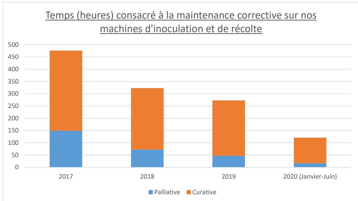
Figure 1: Diagramme de temps dédié à la maintenance corrective sur les machines d'inoculation et de récolte de 2017 à 2020.
