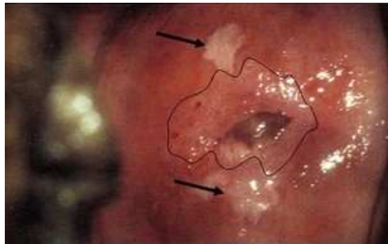
Acide Acétique
