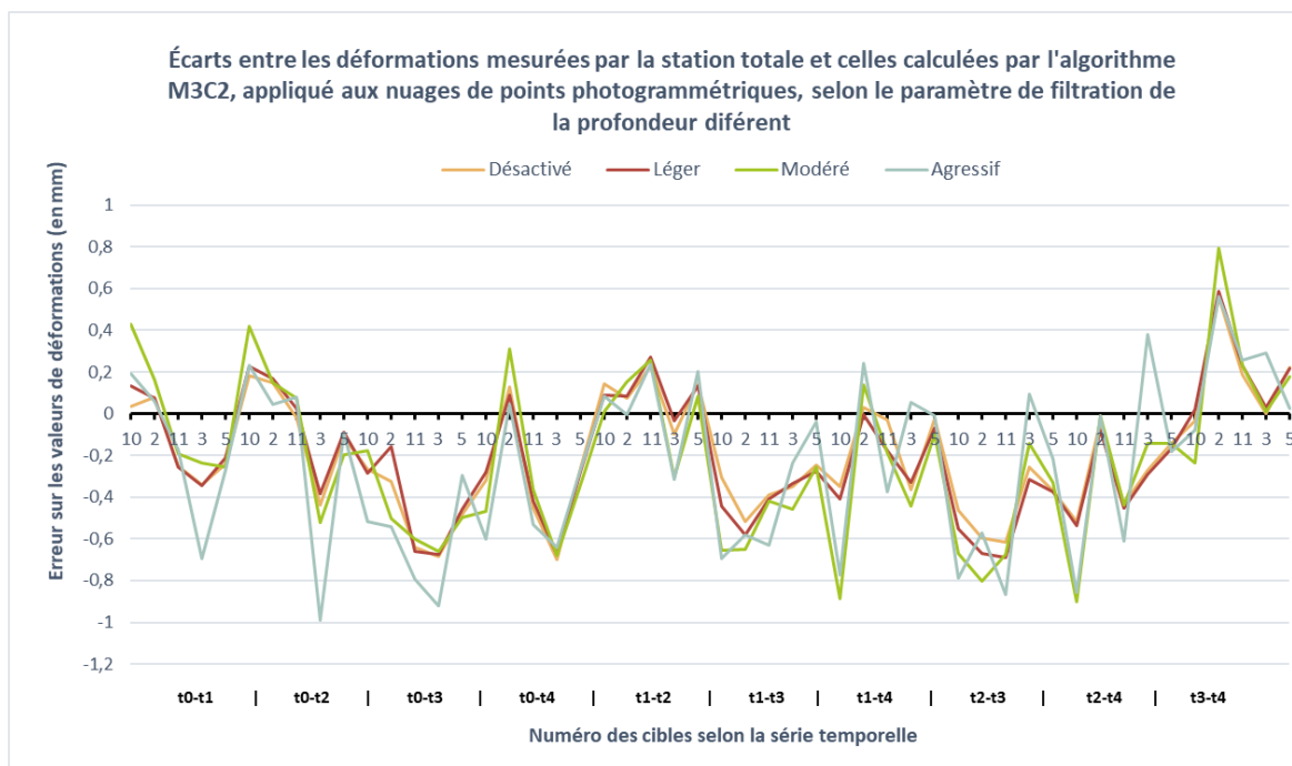
Figure 21 – Graphique des erreurs des déplacements selon le filtre de la profondeur. Auteur : Benoît Brizard
