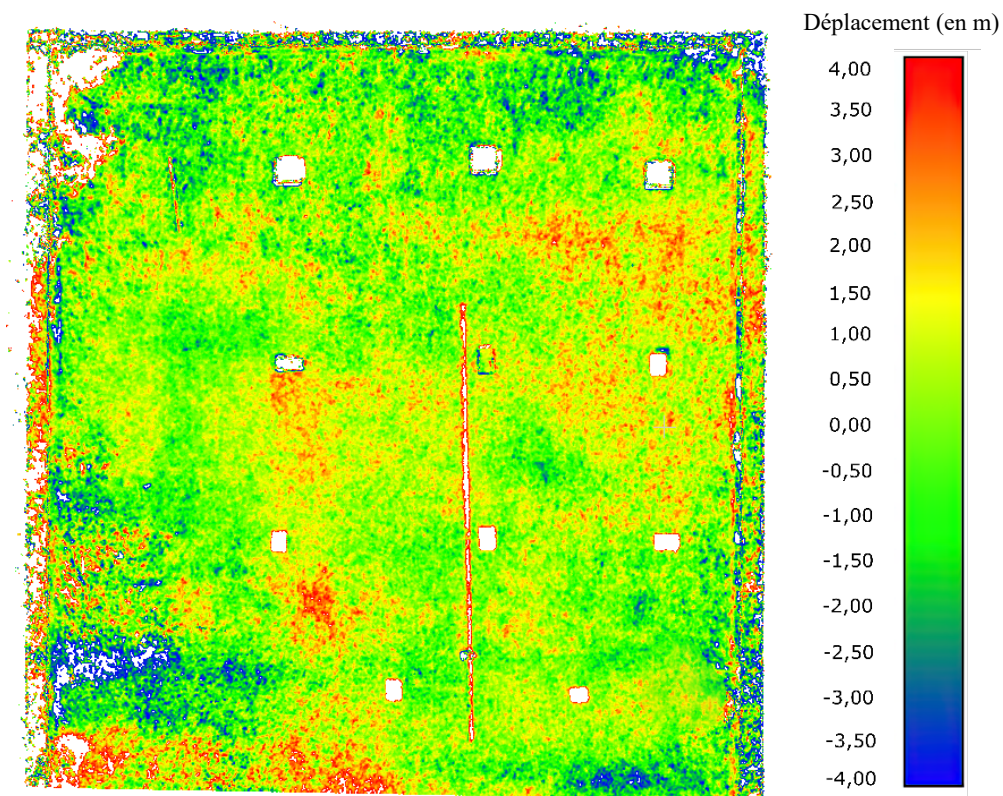
Figure 29 – Cartes des déplacements dont chaque valeur est située dans l'intervalle [-4 mm ; +4 mm]. Auteur : Benoît Brizard
