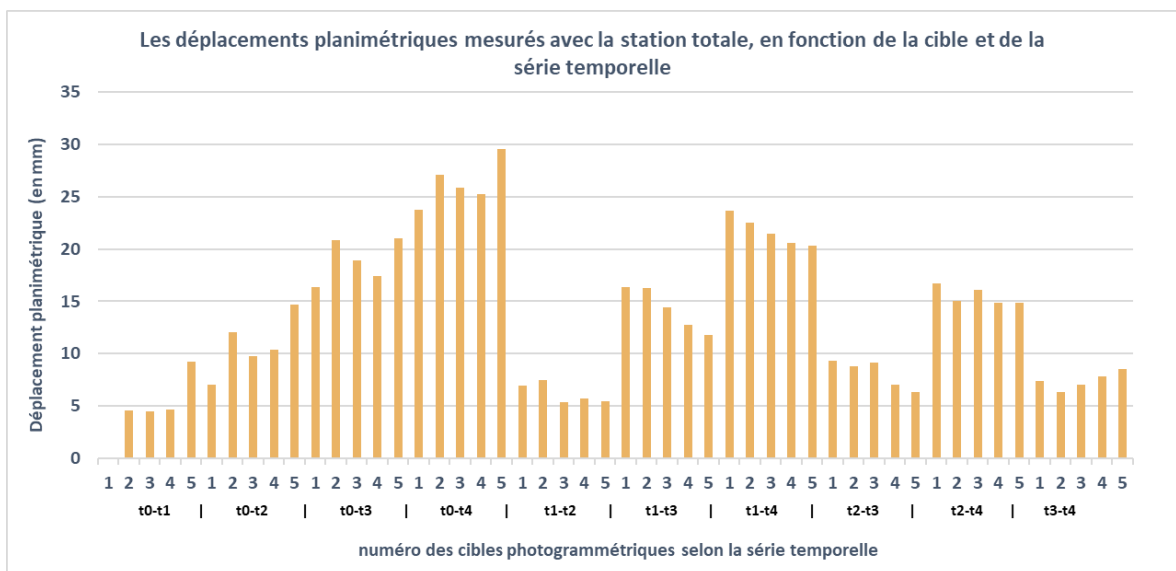
Figure 12 – Graphique des déplacements lors de l'expérience en photogrammétrie terrestre. Auteur : Benoît Brizard
