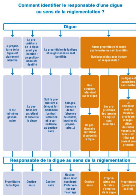
Figure 5 : Le responsable d'une digue au sens de la réglementation ? Source : Les guides du CEPRI, les digues de protection contre les inondations (2010)
