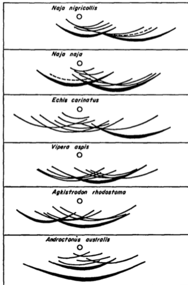
Figure 26 : Exemples d'immunogrammes de venin de serpents et d'un scorpion. [42]
