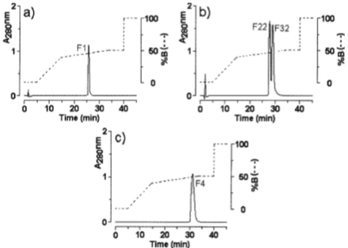
Figure 37 : Résultats de l'HPLC phase inverse réalisée à partir de trois fractions de crotonamines. Fraction IV-3 (figure a), fraction IV-4 (figure b), et fraction IV-7 (figure c). [52]
