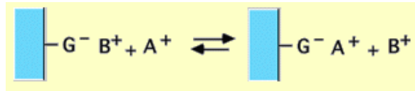
Figure 28 : Schéma simplifié de la réaction d'échange d'ions. [45]
