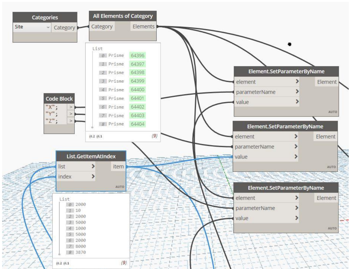
Figure 27: Script pour définir les paramètres XYZ de l'élément (Source personnelle)
