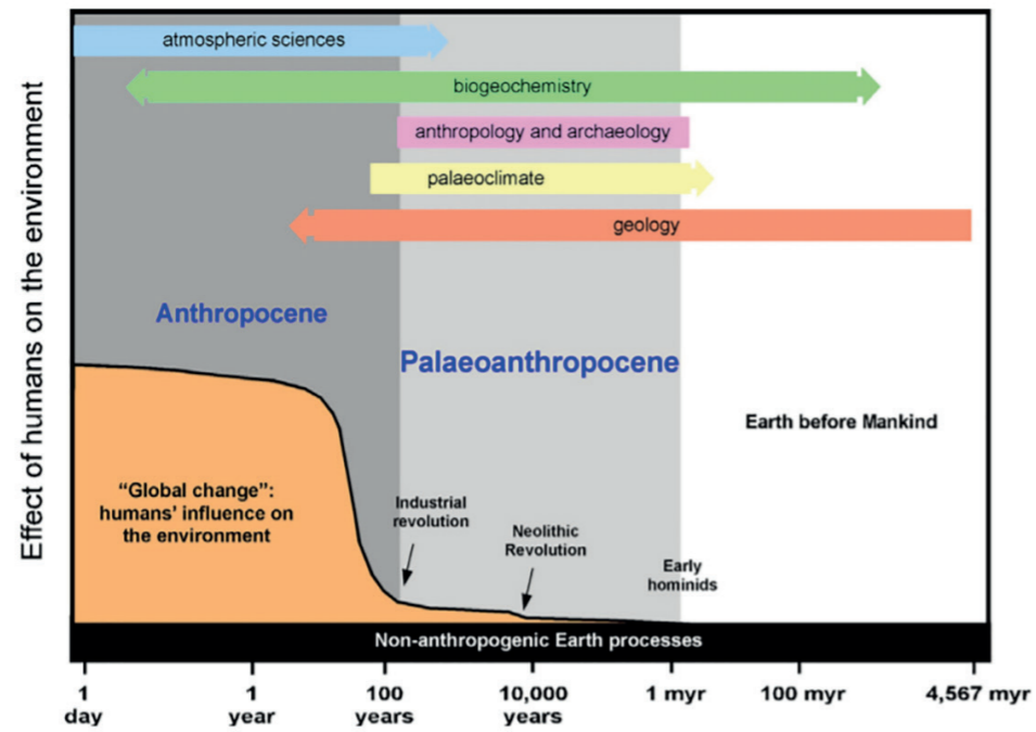
Fig.4: Graphique de Foley. L'histoire de la Terre est placée sur une échelle logarithmique. La paléanthropocène et la période avant l'humanité ont eu peu d'impacts sur l'évolution de la Terre. C'est à la révolution industrielle, donc au commencement de l'anthropocène que les changements globaux se sont fait ressentir. Dans la partie supérieur du graphique, nous pouvons voir les disciplines qui permettent d'étudier chaque période. Il faut noter que les observations de ce schéma restent grandement débattues dans la communauté scientifique.
