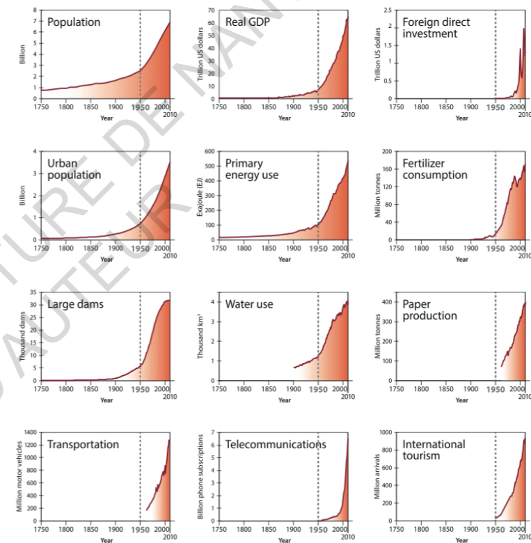
Fig.5: Graphiques produits par l'IGBP, pour illustrer l'évolution des facteurs socio-économiques. Nous pouvons noter une forte augmentation dès l'année 1950.
