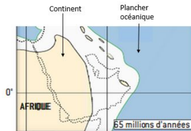
Document 1. Schéma de la surface de la Terre il y a 65 millions d'année au niveau de la plaque Africaine. Les pointillés représentent les limites de la future plaque Arabique.
