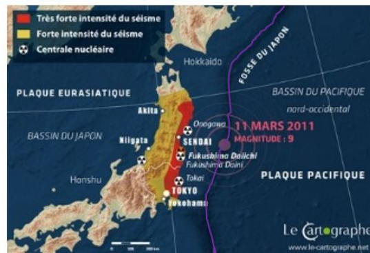
Document 1. Carte de la surface de la Terre au niveau du Japon. L'épicentre* du séisme du 11 mars 2011 est indiqué par un rond violet.
