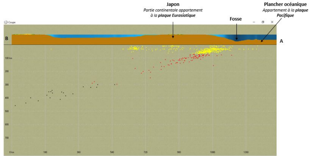
Document 3. Schéma d'une coupe verticale (trait de coupe doc.2) de l'intérieur de la Terre au niveau du Japon
