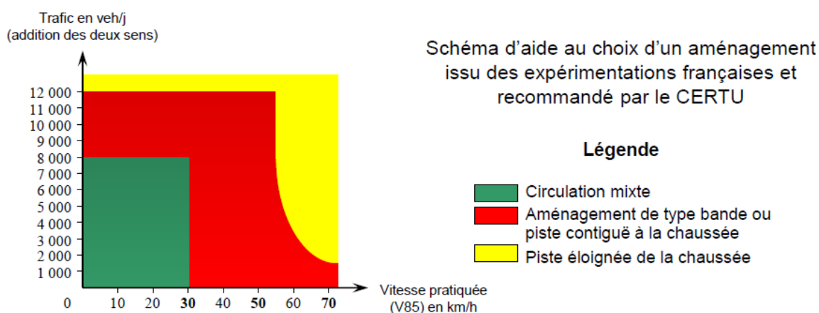
Figure 12: Schéma d'aide au choix d'un aménagement issu des recommandations par le CERTU
