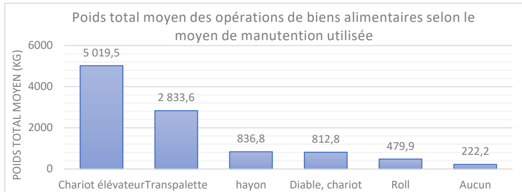
Figure 33 – Poids total moyen des opérations de biens alimentaires selon le moyen de manutention Source : Réalisation personnelle, données issues de l'ETMV Bordeaux 2013
