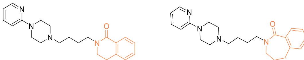
Figure 25: composés obtenus ayant la plus petite affinité pour D2 avec cycles benzolactames en orange
