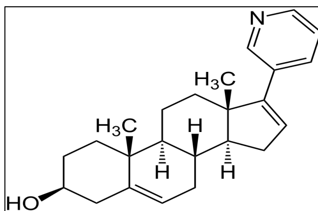
Figure 11. DCI abiratérone (acétate) - Nom UICPA: (3β)-17-(pyridin-3-yl)androst-5,16-dién-3-ol (67)
