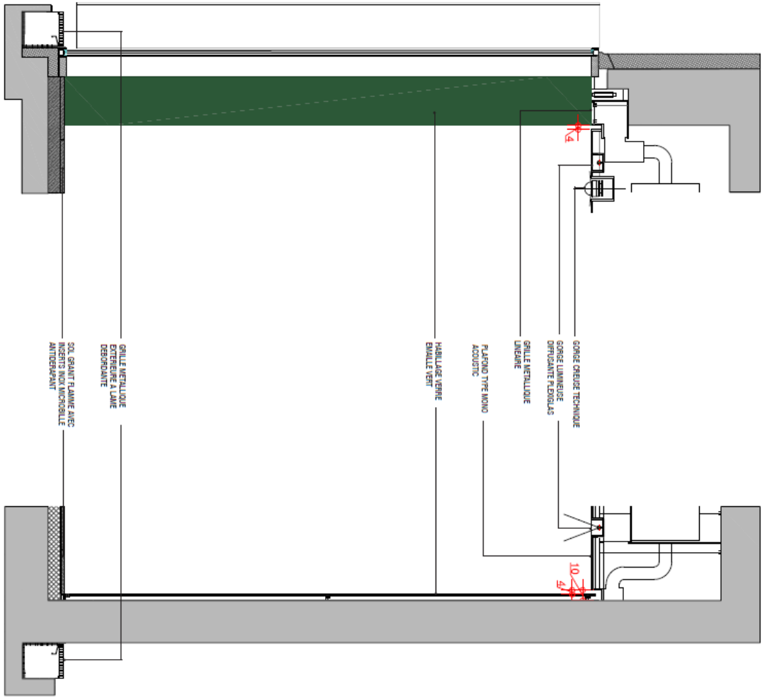
DU02 - Coupe B
