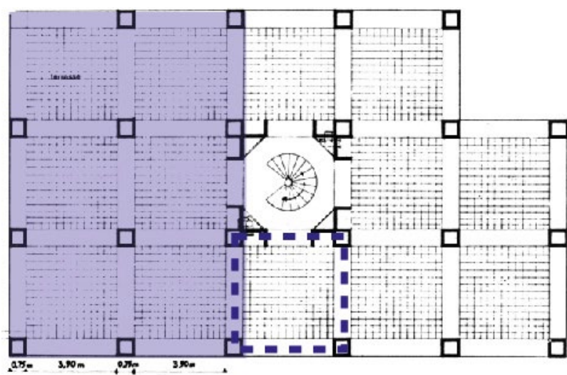
Fig. 19 : plan d'un étage courant, Image retravaillée
