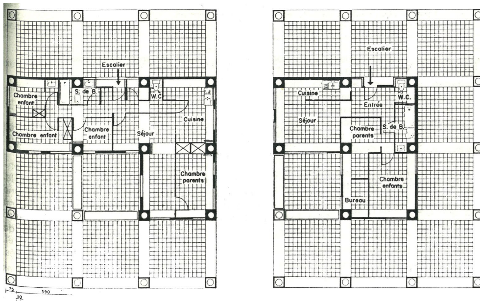
Fig. 18 : plans de différents logements des Marelles
