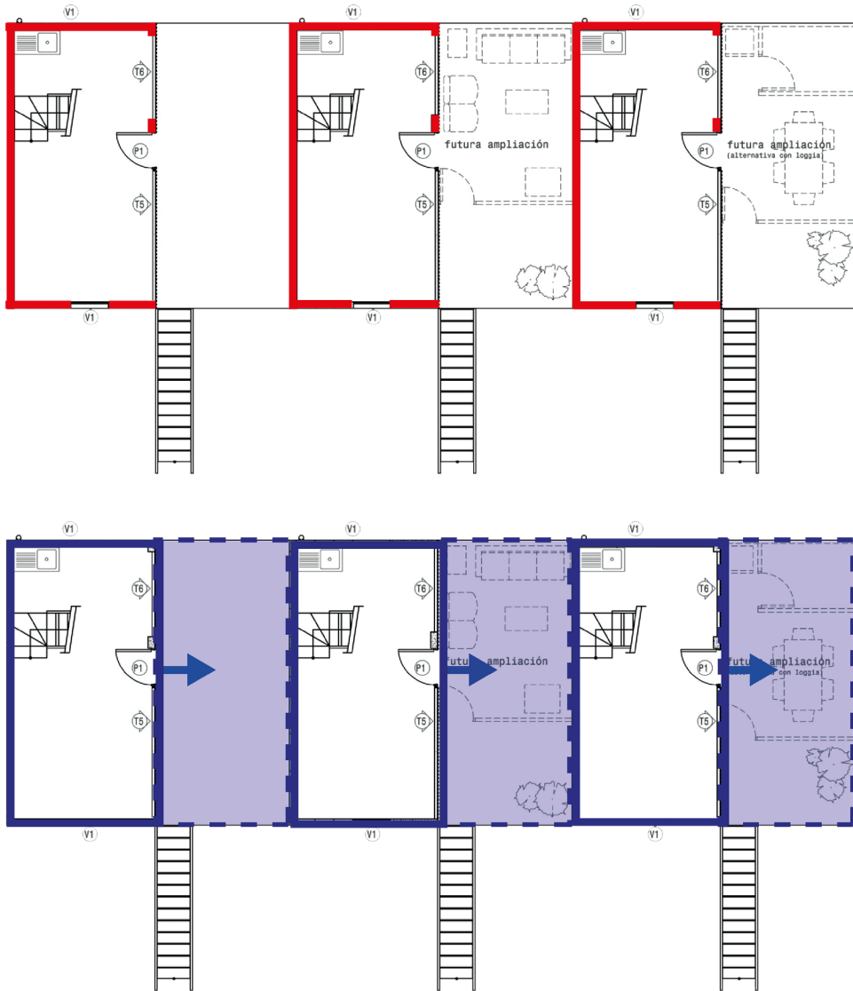
Fig. 35 : plan logement, Image retravaillée
