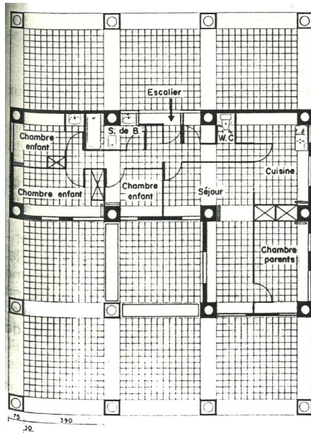
Fig. 18 : plans de différents logements des Marelles
