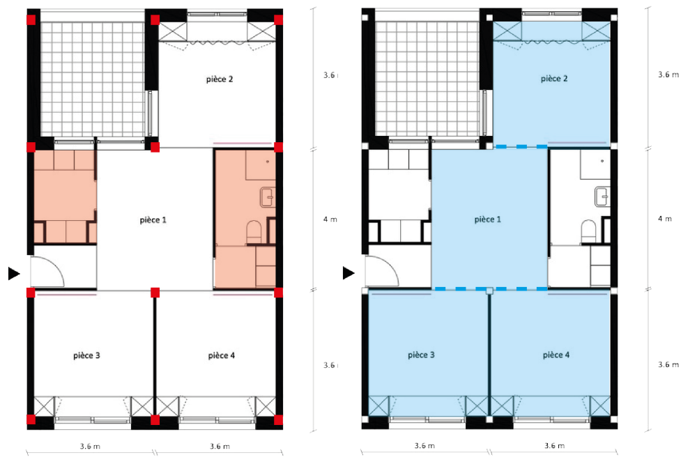
Fig. 30 : plan d'un logement, Image retravaillée
