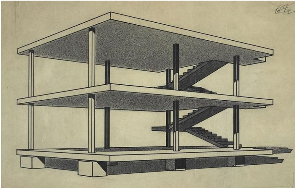
Fig. 7 : dessin de la maison Dom-ino
