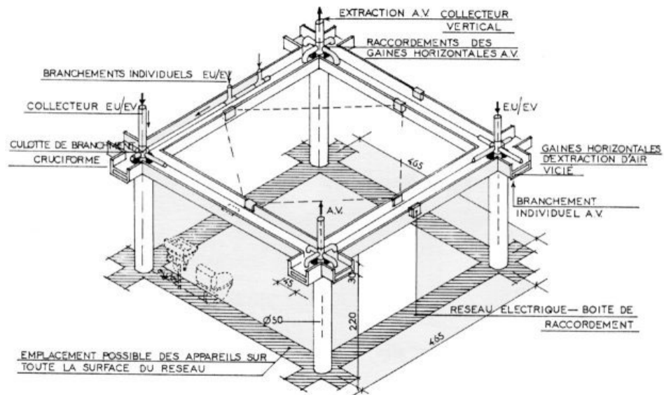
Fig. 17 : schéma de la structure poteaux-poutres des Marelles
