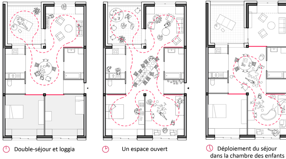
Fig. 29 : plans de différentes appropriations possibles dans un même logement
