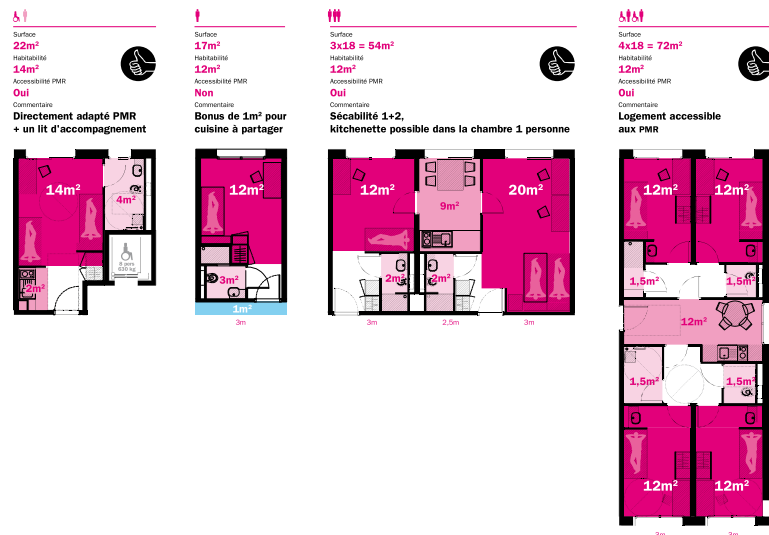
Fig. 46 : Proposition de logements par Canal Architecture
