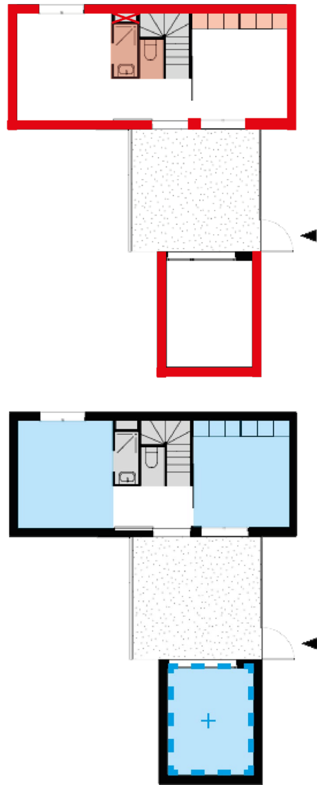
Fig. 25 : plan d'un logement, Image retravaillée
