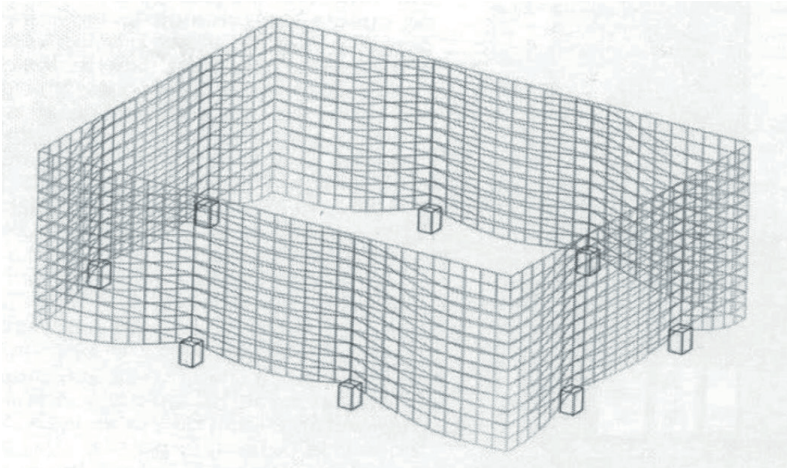
fig.31 : La Ferriera, Locarno, axonométrie structurale de la façade, 2003
