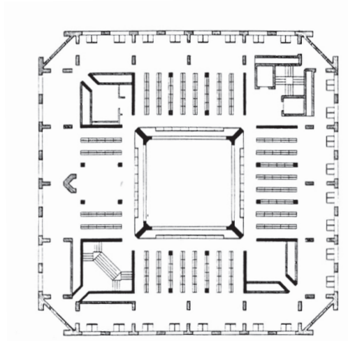
fig.25 : Bibliothèque académique Exeter, New Hampshire, Louis Kahn, plan d'étage, 1965-1972
