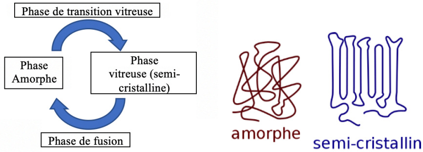
Figure 13 : Schéma des différentes phases de transition d'un polymère thermo-plastique.
