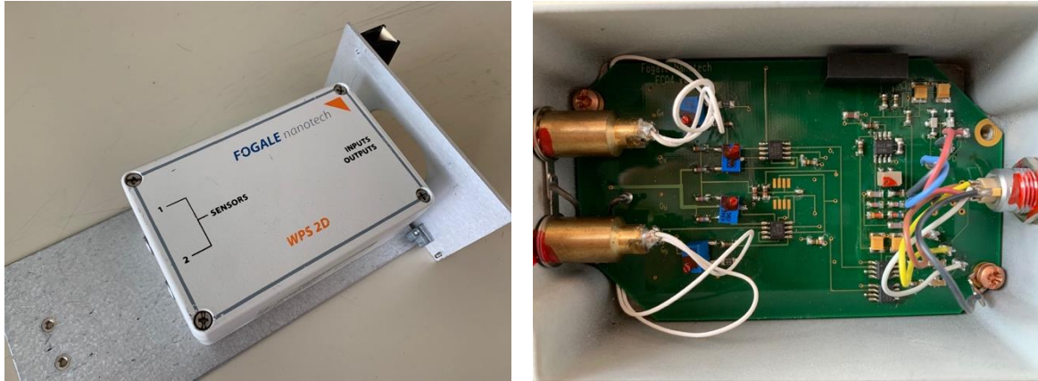
FIG. 4 — Conditionneur de marque Fogale Nanotech. Le circuit électronique est placé dans un boîtier hermétique. Le capteur est relié par une paire de câbles et le conditionneur est relié au système d'acquisition par un unique câble.
