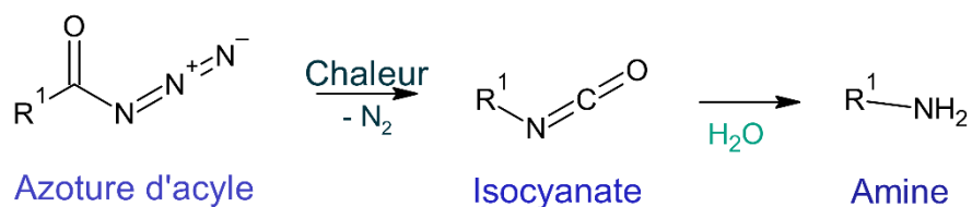
Figure 3 - Réaction de Curtius
